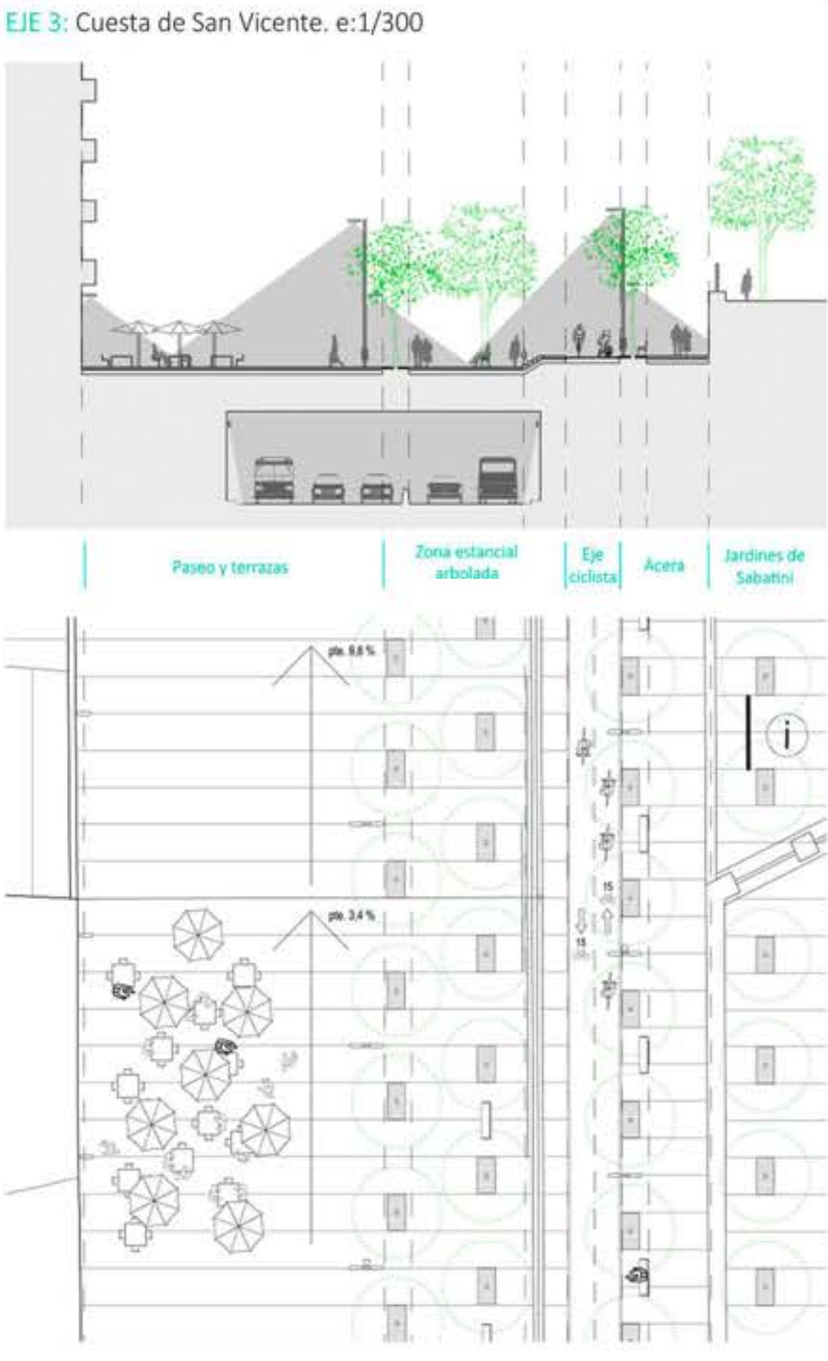
EJE 3: Cuesta de San Vicente. e:1/300
