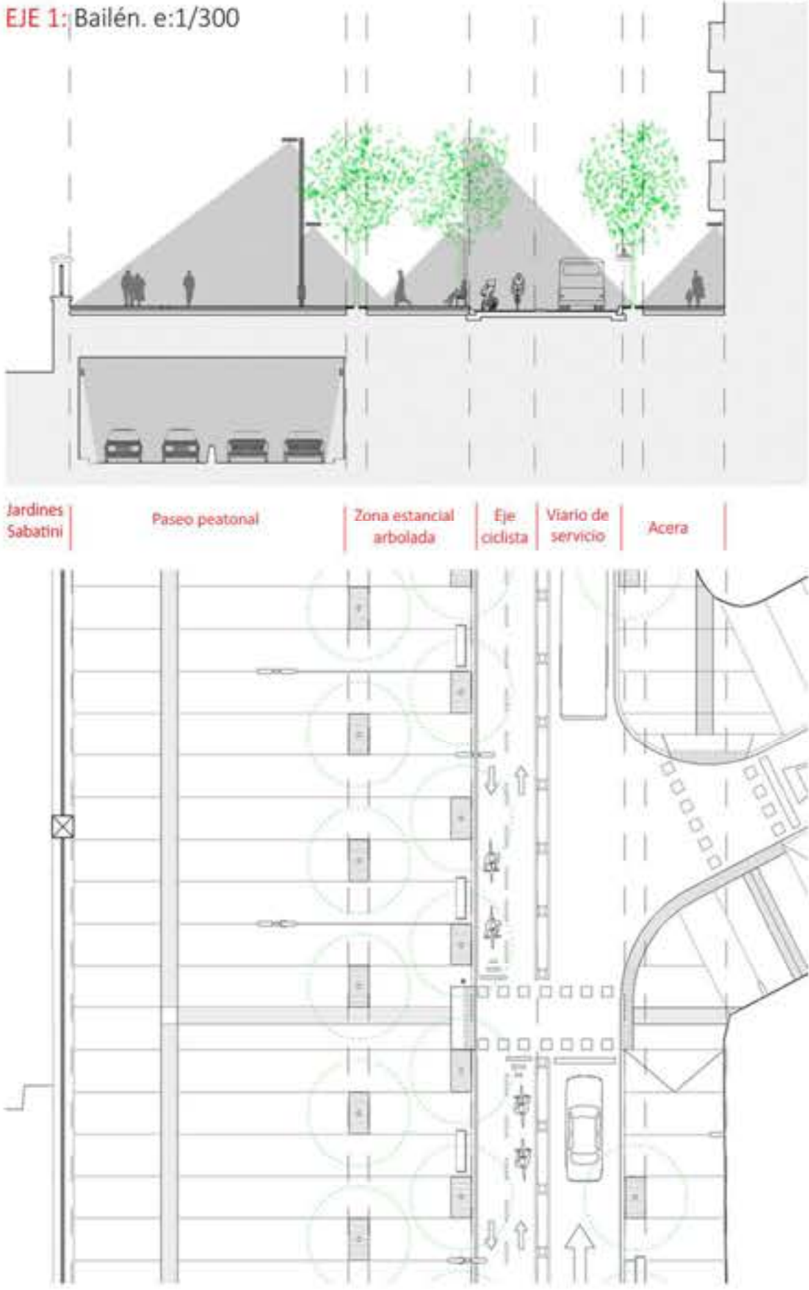
EJE 1: Bailén. e:1/300
