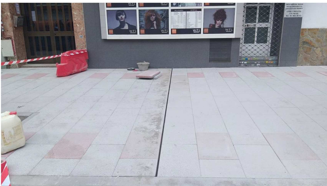
Fotografía 3.- Calle Castrojeriz entre Nº 14 y Nº 12: Detalle de la junta de dilatación del solado, dispuestas cada 20 metros.
