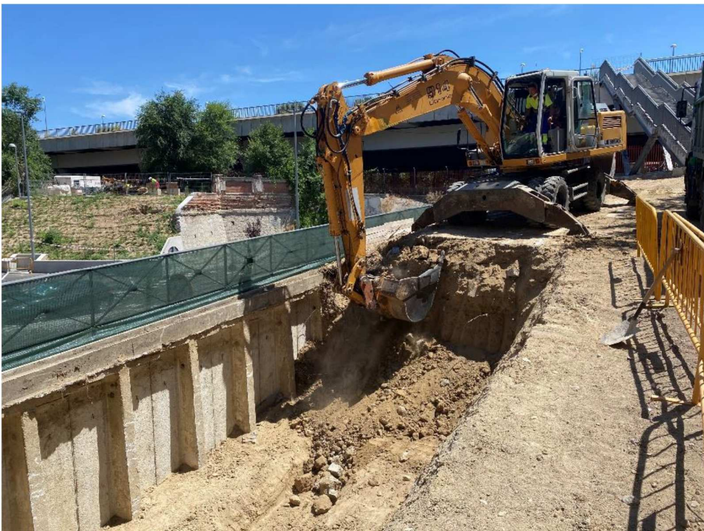
Foto 2: Labores de excavación en el trasdós del muro
